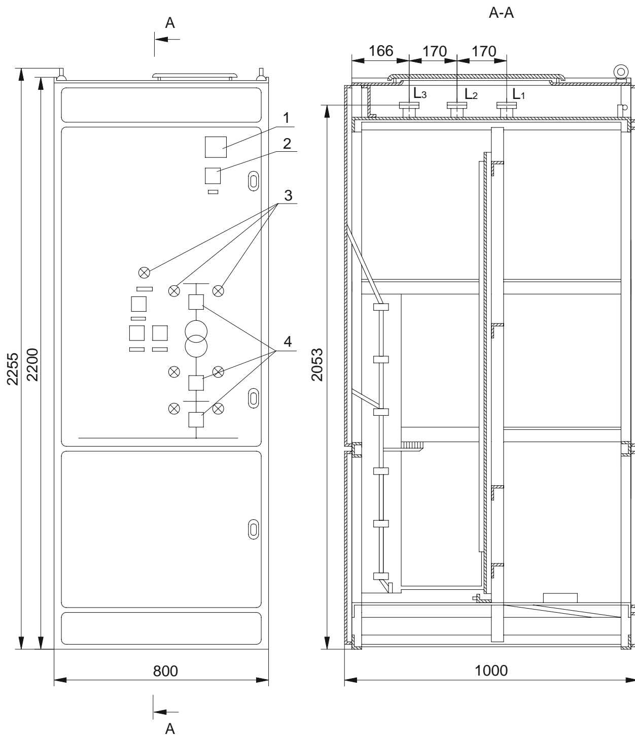
Рис. 24 Габаритные размеры шкафов 7ШН-70 (5ШН-70): 1 - амперметр, 2 - указательное реле, 3 - сигнальные лампы, 4 - переключатели.
