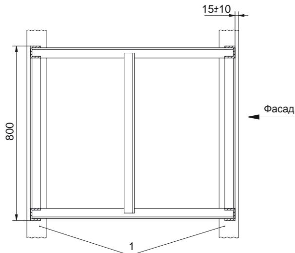
Рис. 10 Установочные размеры шкафов 8ШН-10 7ШН-12К, 7ШН-13С: 1 - закладной швеллер (в поставку завода не входит). Сварной шов прерывистый.
