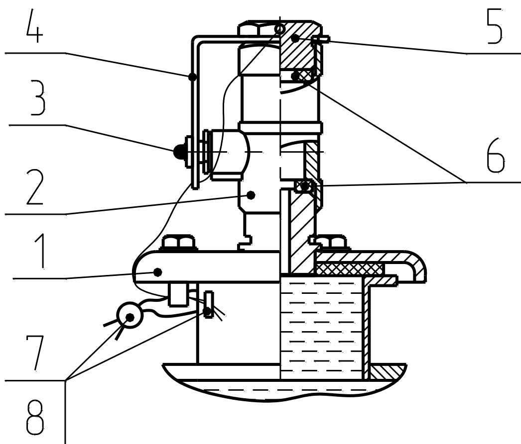
1 - крышка патрубка; 2 - кран шаровой; 3- винт; 4 - ручка крана; 5 - пробка; 6 - резиновая прокладка; 7 - проволока; 8 - пломба
