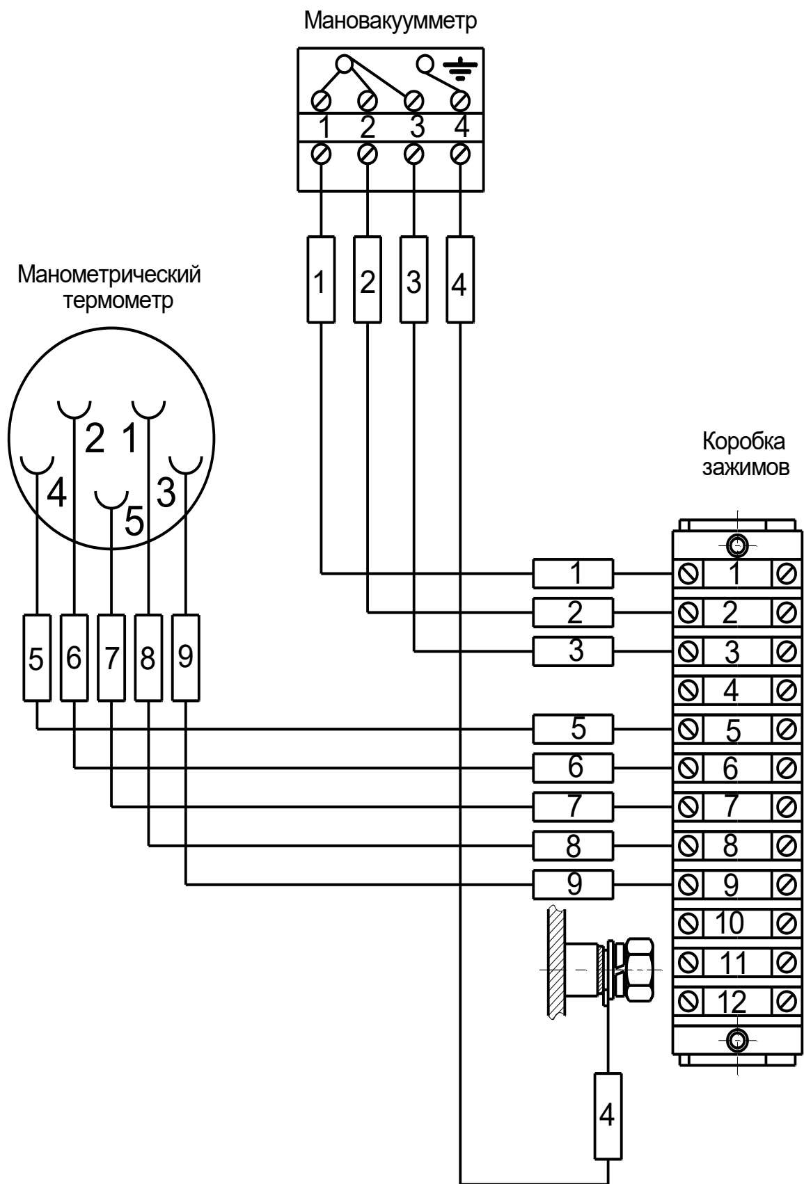
Рисунок А.17 – Монтажная схема соединения коробки зажимов с контрольно-измерительными приборами
