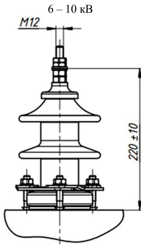
Рисунок А.5 – Вводы ВН
