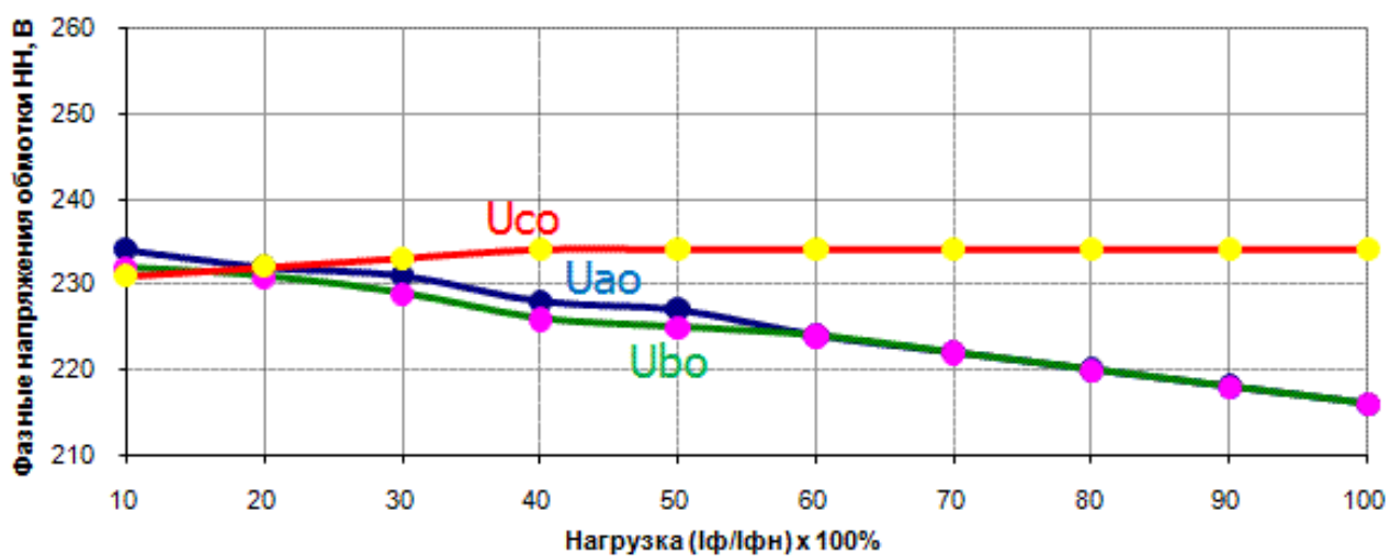
ТМГСУ-25/10-У, 10/0,4 кВ, У/Ун-0, двухфазная нагрузка (а-0 и b-0)
